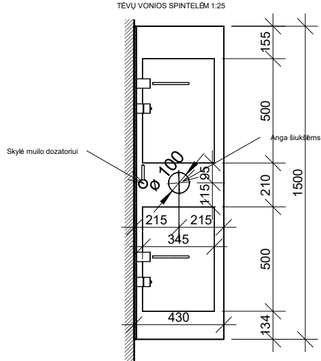
VAIZDAS PLANE M1:25
