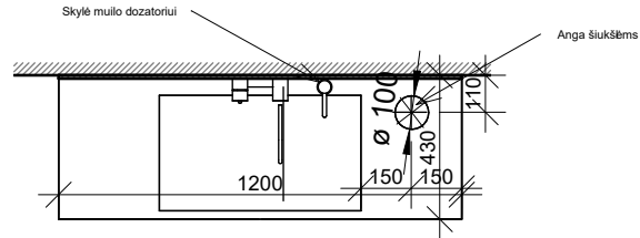
VAIZDAS PLANE M1:25
