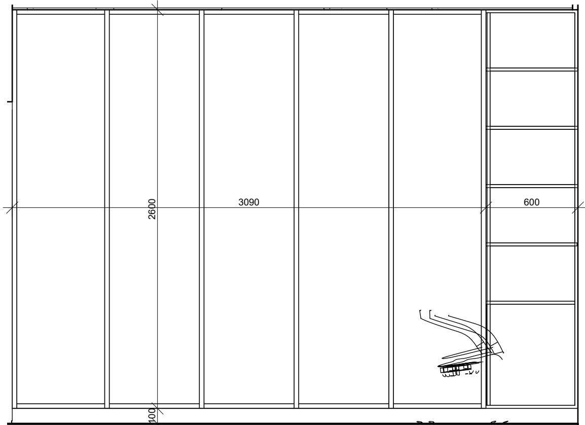
Spinta gaminama stiklinėmis, stumdomomis durimis, rėmo spalva RAL 7016
