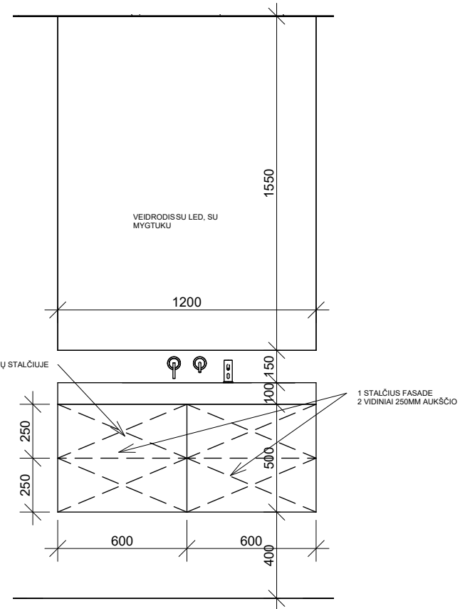
VAIZDAS IŠ PRIEKIO M 1:25
