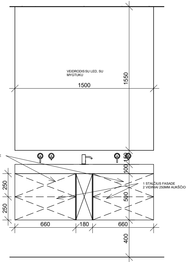
VAIZDAS IŠ PRIEKIO M 1:25
