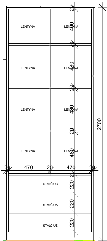
VIDAUS IŠDĖSTYMAS M 1:25
