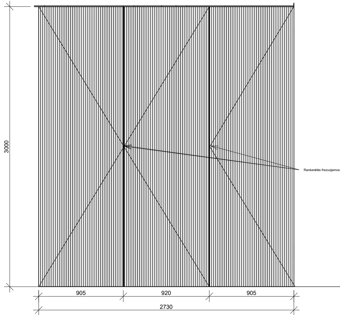
SPINTOS VAIZDAS IŠ PRIEKO M 1:25
