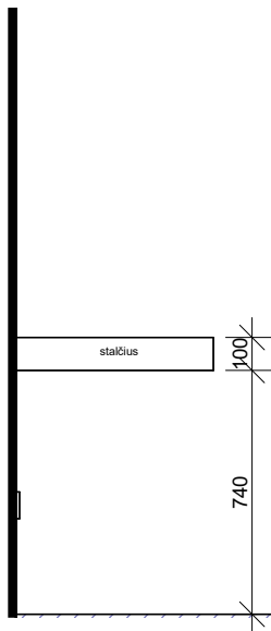
LENTYNĖLĖS VAIZDAS IŠ PRIEKO M 1:25
