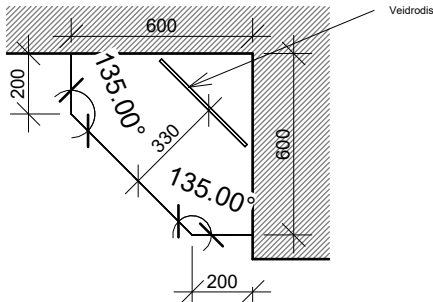
VAIZDAS PLANE M 1:25
