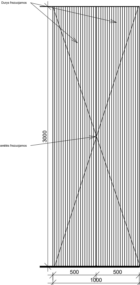
VAIZDAS IŠ PRIEKIO M 1:25
