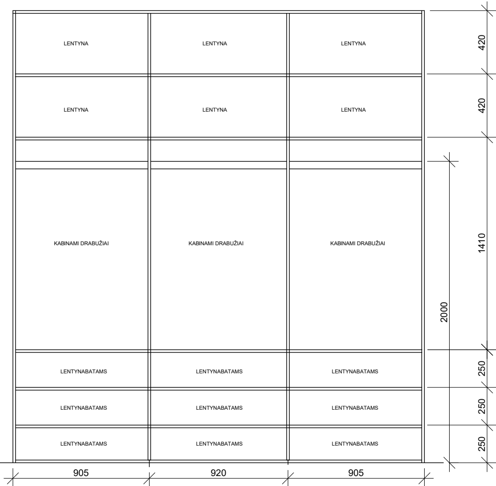
SPINTOS VIDUS M 1:25
