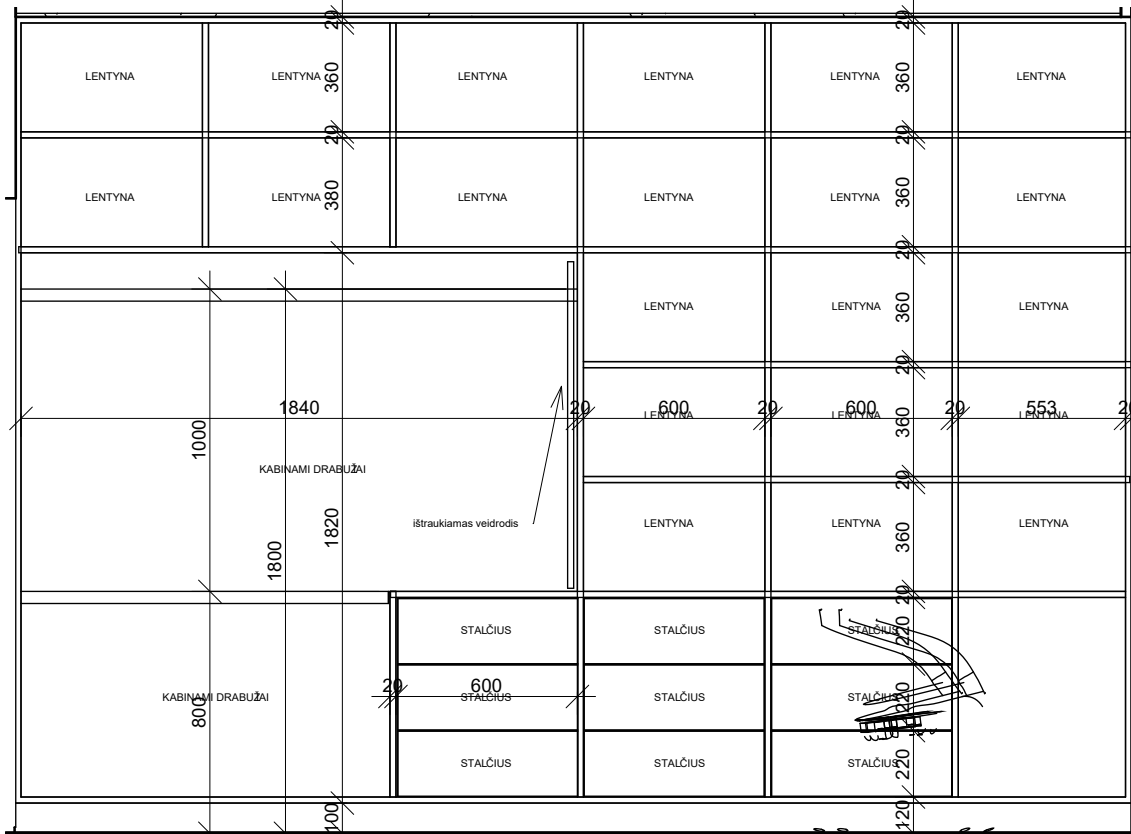
VIDAUS IŠDĖSTYMASM 1:25
