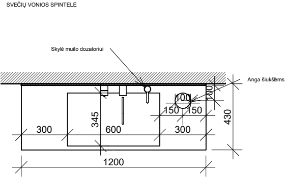
VAIZDAS PLANE M1:25
