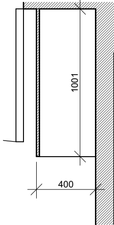
VAIZDAS PLANE M 1:25
