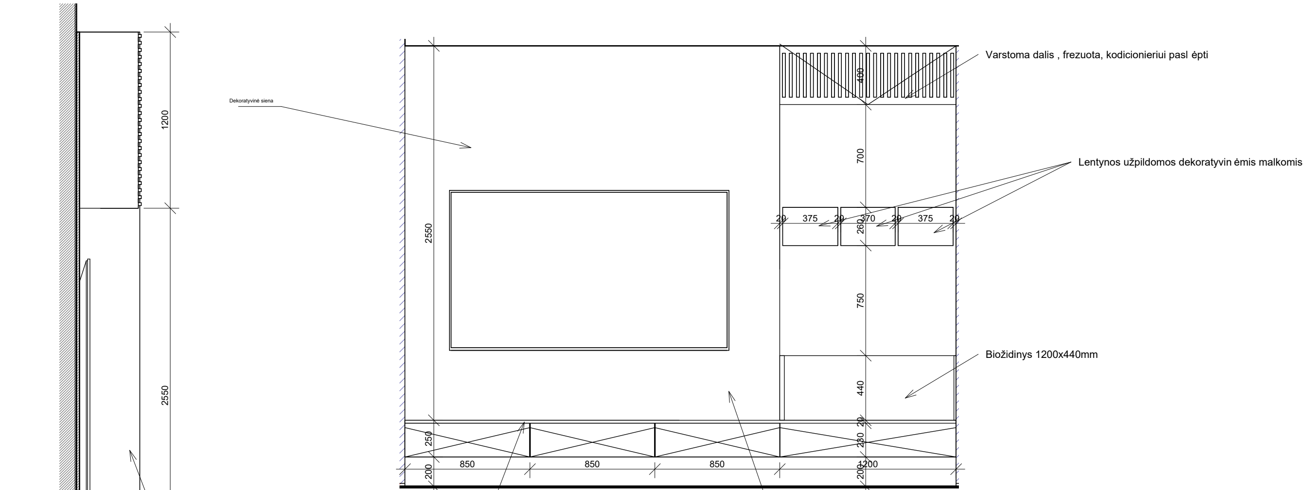
VAIZDAS IŠ PRIEKIO M1:25
