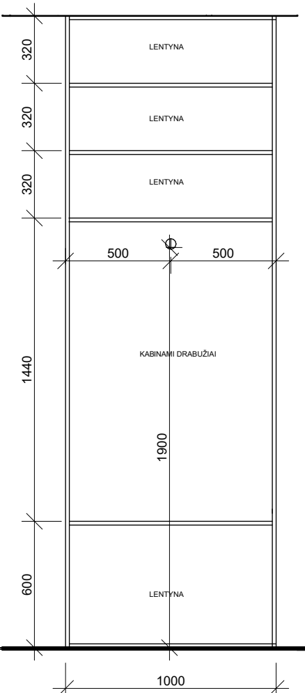
VIDAUS IŠDĖSTYMAS M 1:25
