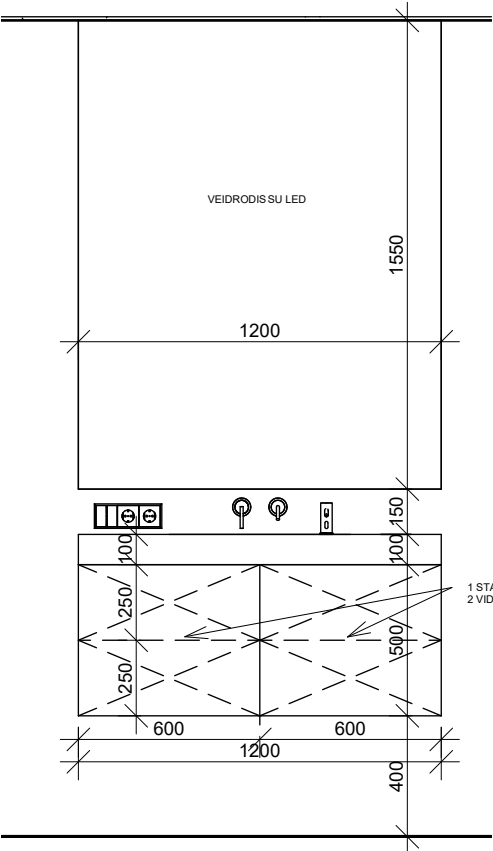
VAIZDAS IŠ PRIEKIO M 1:25
