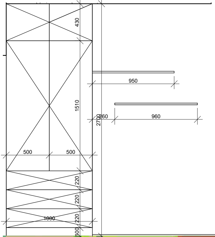
VAIZDAS IŠ PRIEKIO M 1:25
