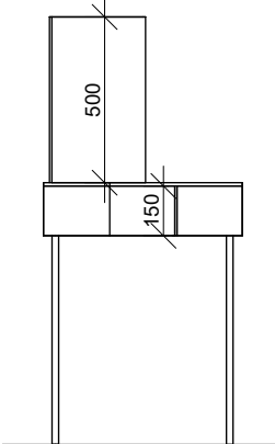
VAIZDAS IŠ ŠONO M 1:25
