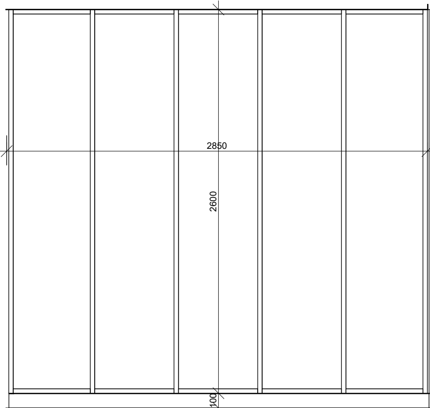
Spintos gaminamos stiklinėmis, stumdomomis durimis, rėmo spalva RAL 7016 VAIZDAS IŠ PRIEKIOM 1:25
