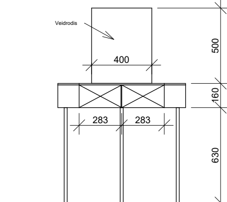
VAIZDAS IŠ PRIEKIO M 1:25
